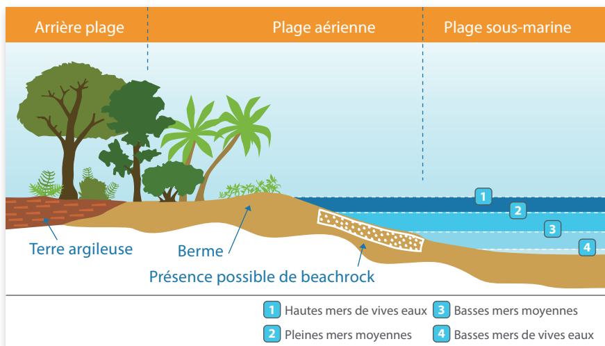
Morphologie et transits sédimentaires d'une plage.
