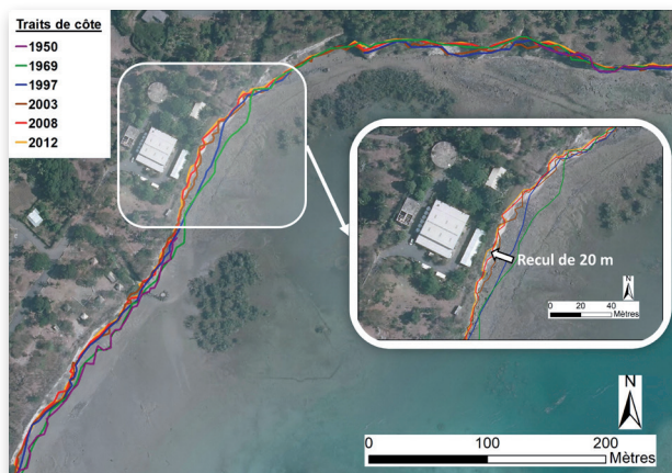
Recul de la falaise de Pamandzi de 1950 à 2012.
